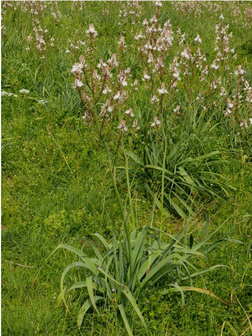
Asphodelus ramosus
